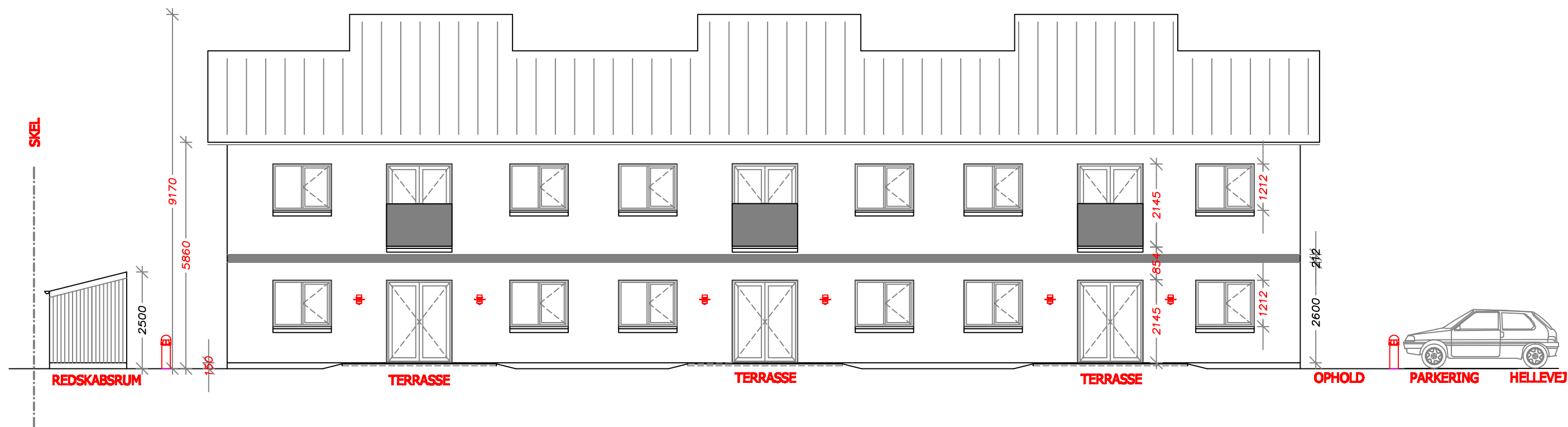
FACADE BYGNING 1 MOD HUNDIGE STRANDVEJ ( VEST )
